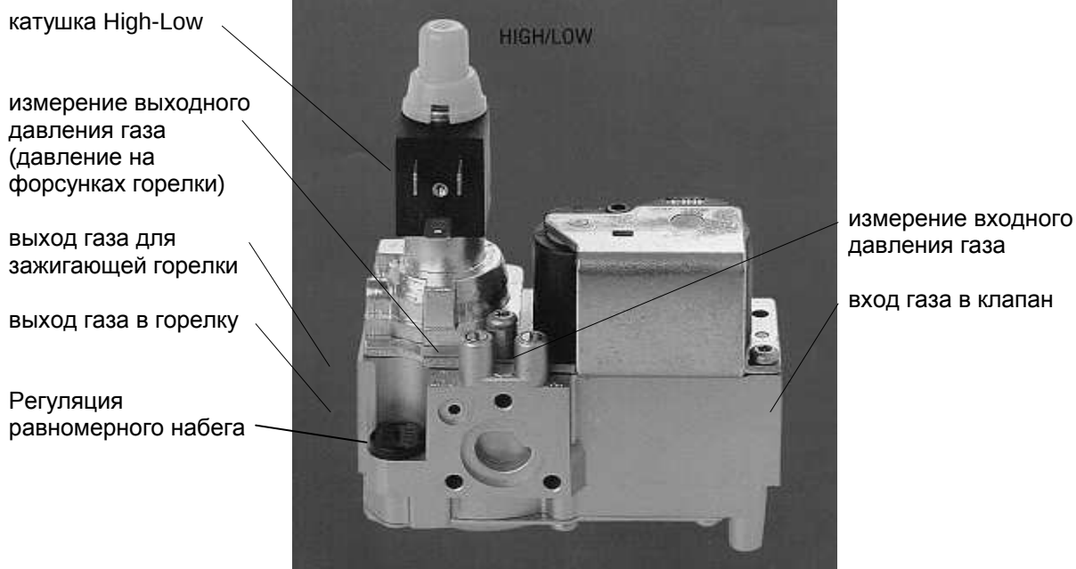
Рис. 25a) Газовый клапан Honeywell VK 4100 Q 2003
