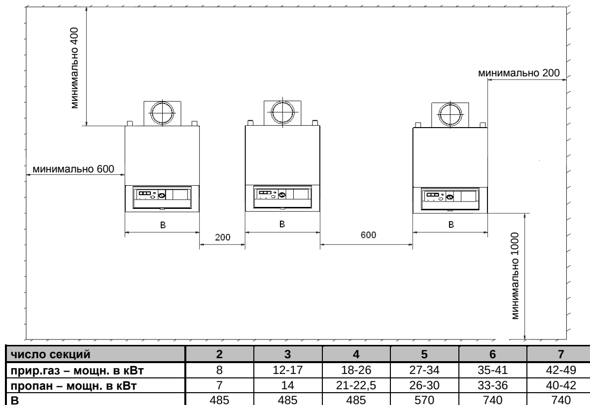
Рис. 17 Расположение котлов в котельной
