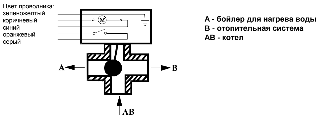
Рис. 21 Трехходовой клапан Honeywell V 4044F
