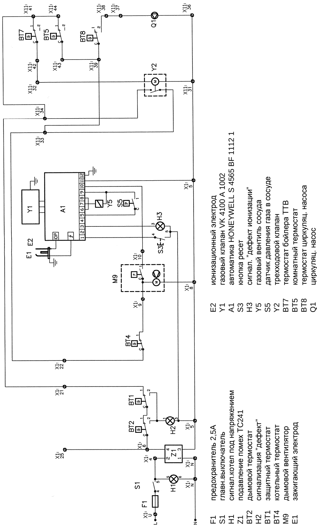
Рис. 9а) Контурная схема включения котла VIADRUS GARDE G 42 и VIADRUS GARDE G 42 ECO для пропана
