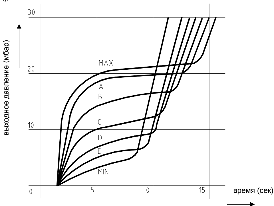
Рис. 27 Характеристики открытия главного клапана
